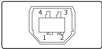
USB "B" 타입
